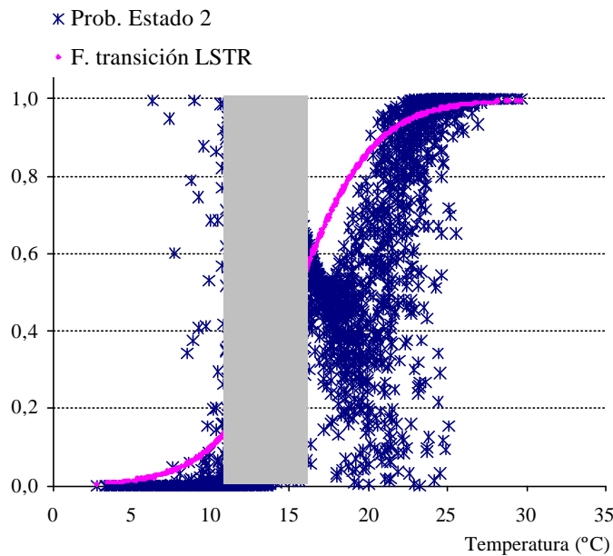
Gráfico 8.- Probabilidad estado 2 y función de transición LSTR estimada vs. Temperatura.
