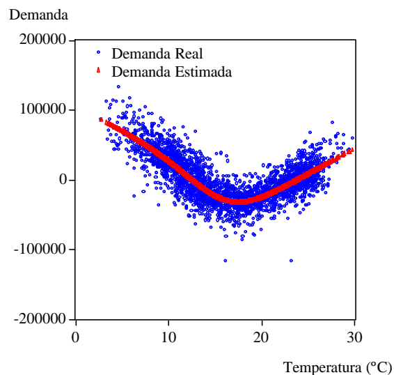
Gráfico 6.-Curva de respuesta real y estimada
