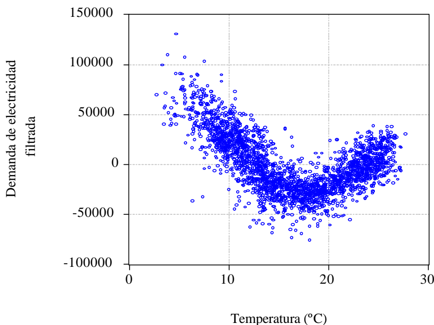
Gráfico 2.- No linealidad de la respuesta de la demanda de electricidad.
